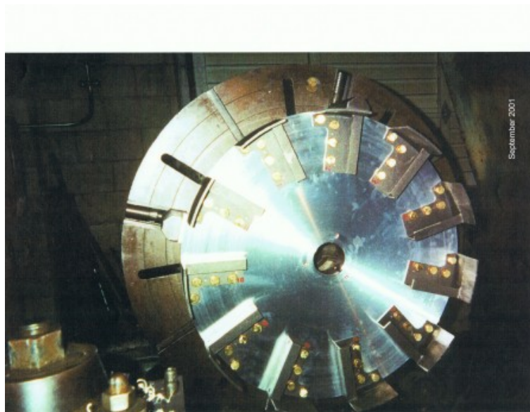
Photographie de pièce du fluxomatic de Lloyd Zirbes.
