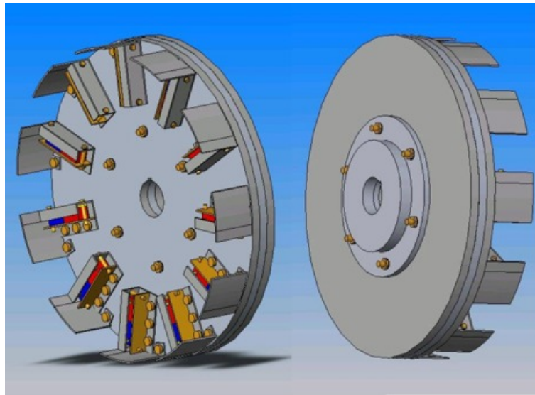
Schéma des pièces du fluxomatic réalisé par Lloyd Zirbes et son équipe Stardust.
