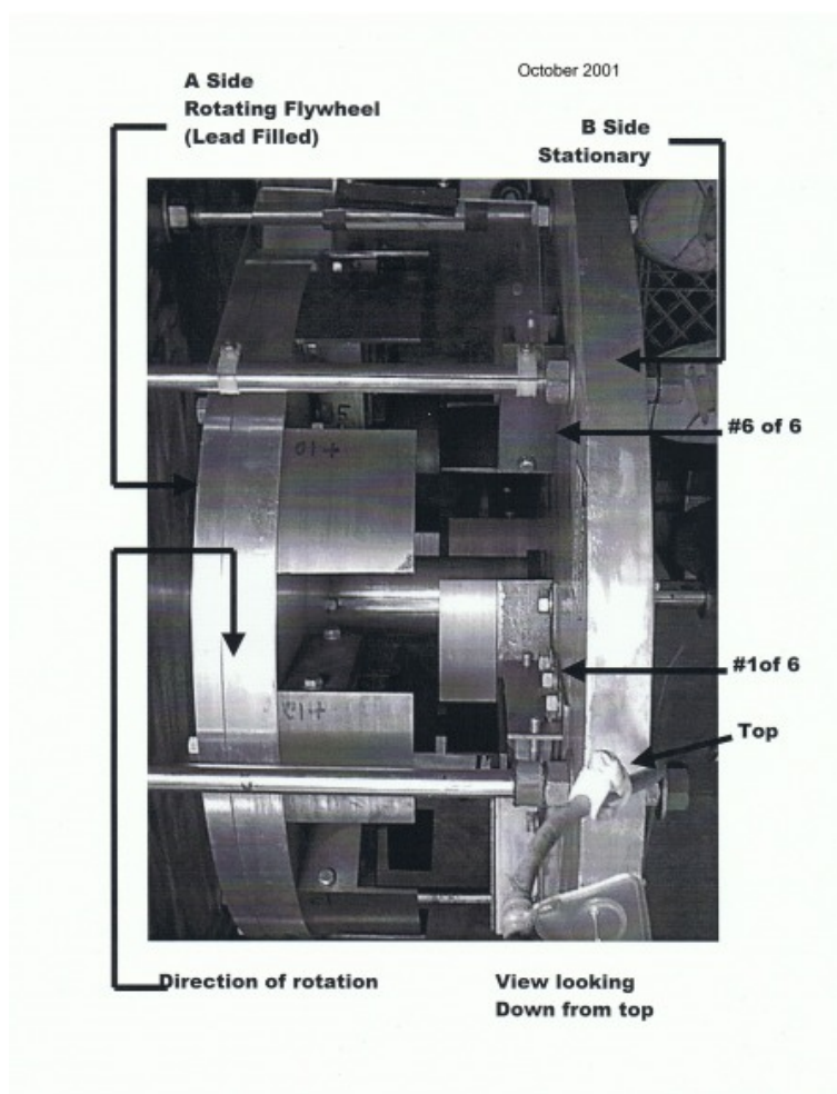
Photographie du fluxomatic complet de Lloyd Zirbes.
