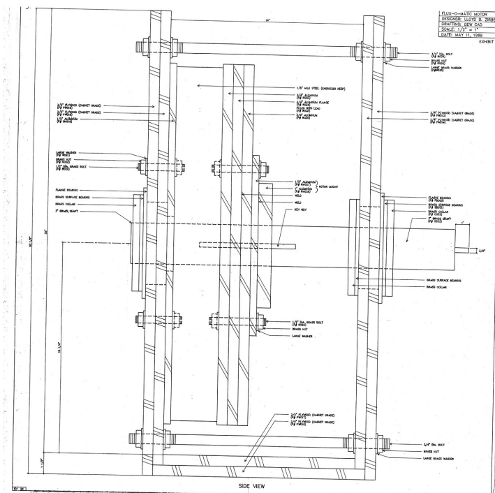
Schéma détaillé de montage du fluxomatic extrait des nombreux schémas disponibles sur le GitHub.
