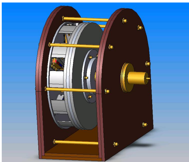
Schéma du fluxomatic réalisé par Lloyd Zirbes et son équipe Stardust.
