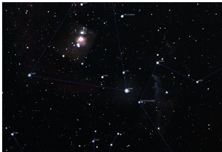
Zoom sur l'étoile Rigel (étoile Beta Orion), qui est en fait un système d'au moins 4 étoiles visibles
