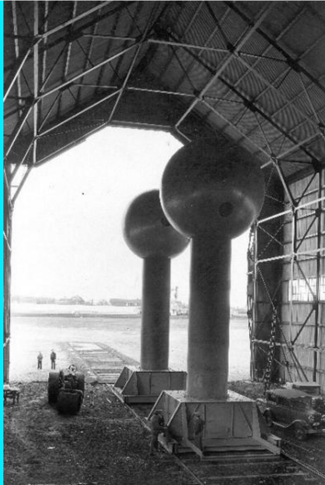
Les deux générateurs de Van de Graaf géants du musée des sciences de Boston, hauts de 7,60 mètres.
