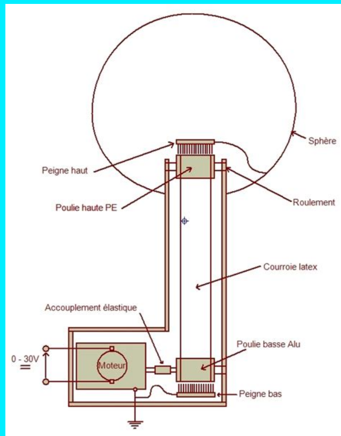
Schéma explicatif d'un générateur de Van de Graaff
