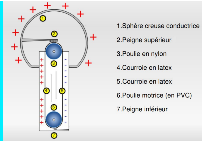
Circulation des charges électrostatiques dans le générateur de Van de Graaf
