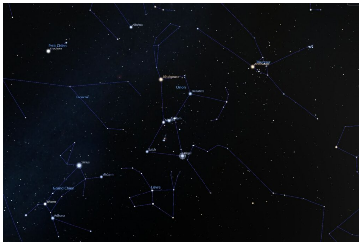
Situation de Rigel dans la constellation d'Orion
